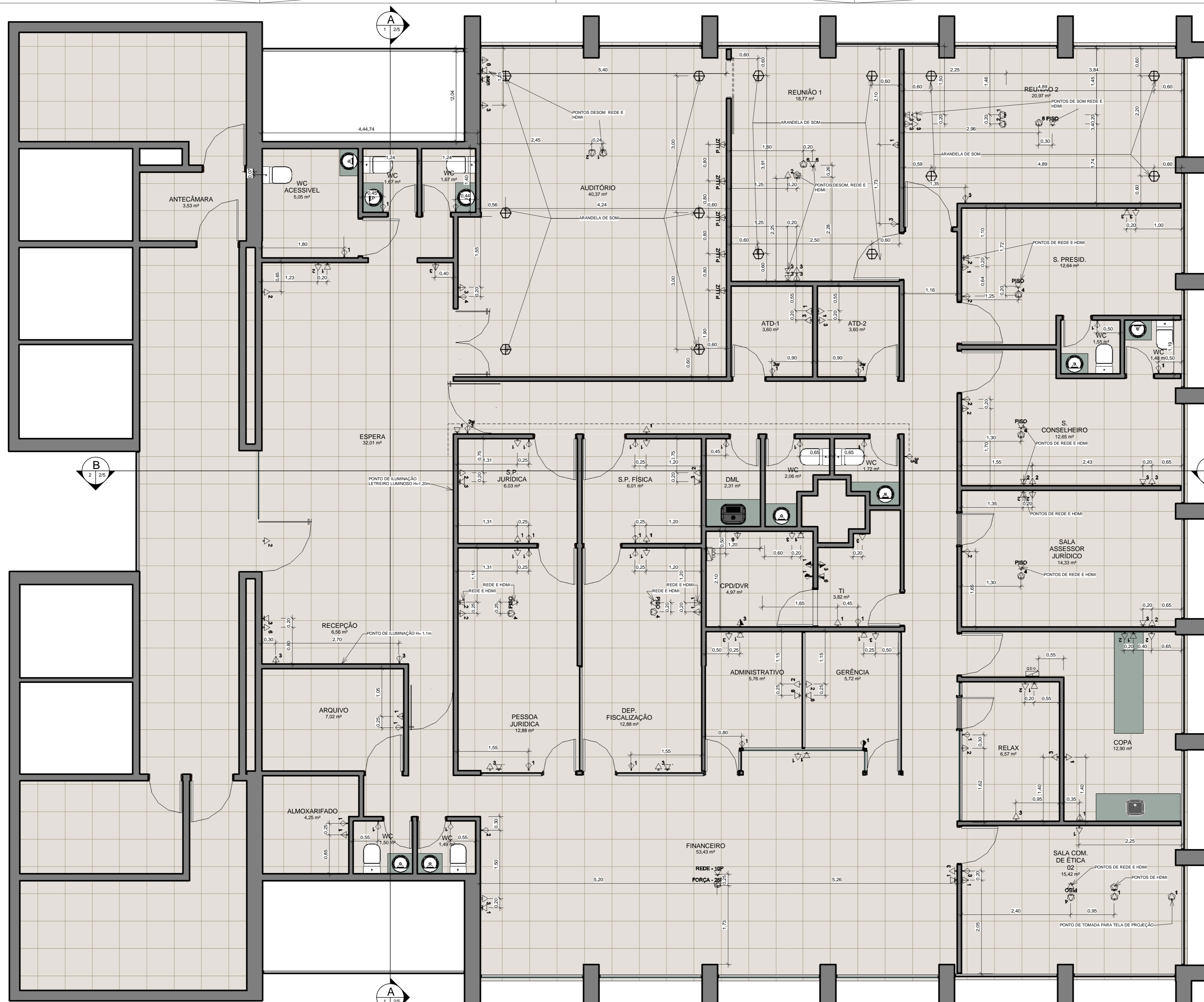
1 PLANTA ELETRICA ESCALA 1 : 50
